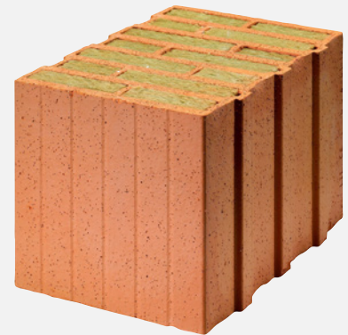
Grossblockstein mit mineralischem Dämmstoff
