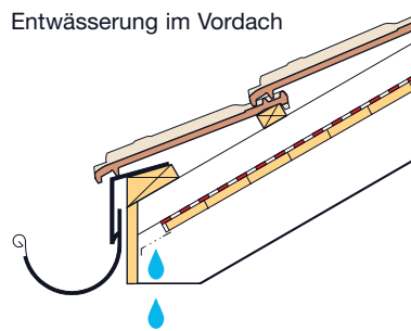
Entwässerung im Vordach
