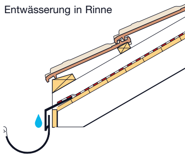
Entwässerung in Rinne
