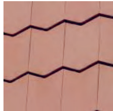
Biberschwanzziegel Einfachdach Lattweite: ca. 22 – 23 cm Deckbreite: ca. 17 cm Ziegelbedarf: ca. 25 Stk./m 2
