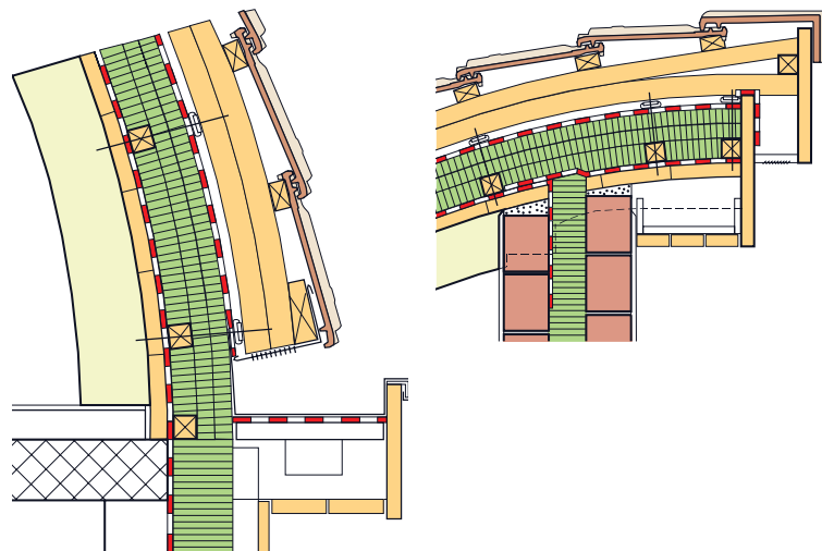
Traufe mit Kastenrinne
