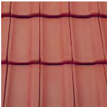
Flachziegel (Jura-Ziegel) Lattweite: ca. 32 – 37 cm Deckbreite: ca. 21 – 22 cm Ziegelbedarf: ca. 13 Stk./m 2
