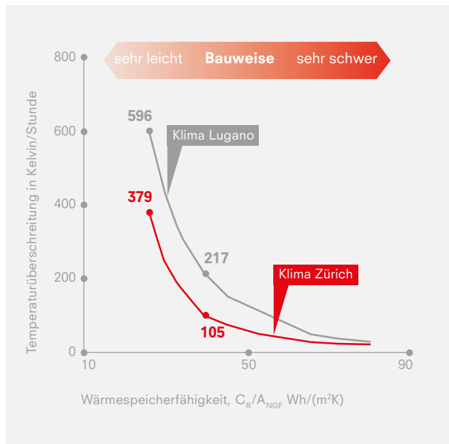
Abbildung 2: Überschreitung der zulässigen Raumtemperatur in Funktion der Wärmespeicherfähigkeit
