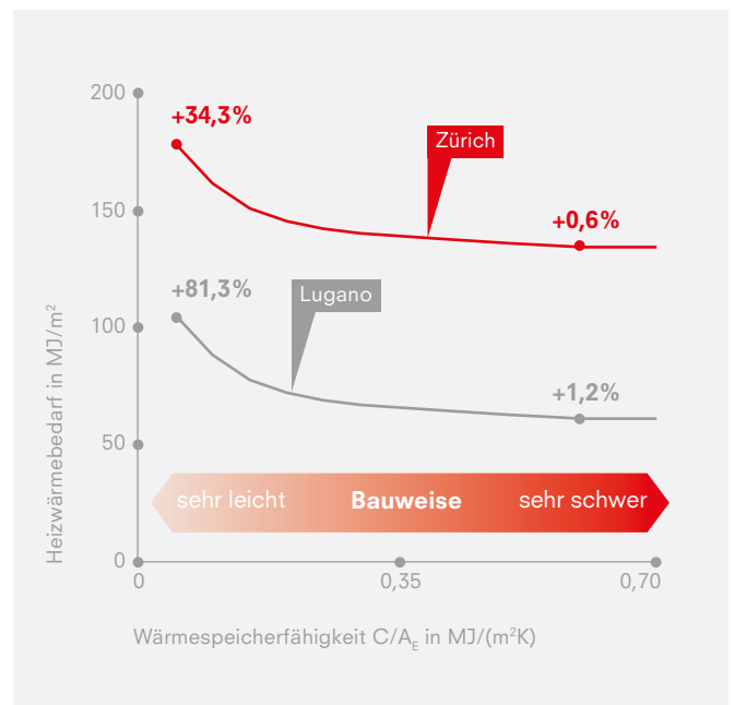
Abbildung 1: Einfluss der Wärmespeicherfähigkeit auf den Heizwärmebedarf
